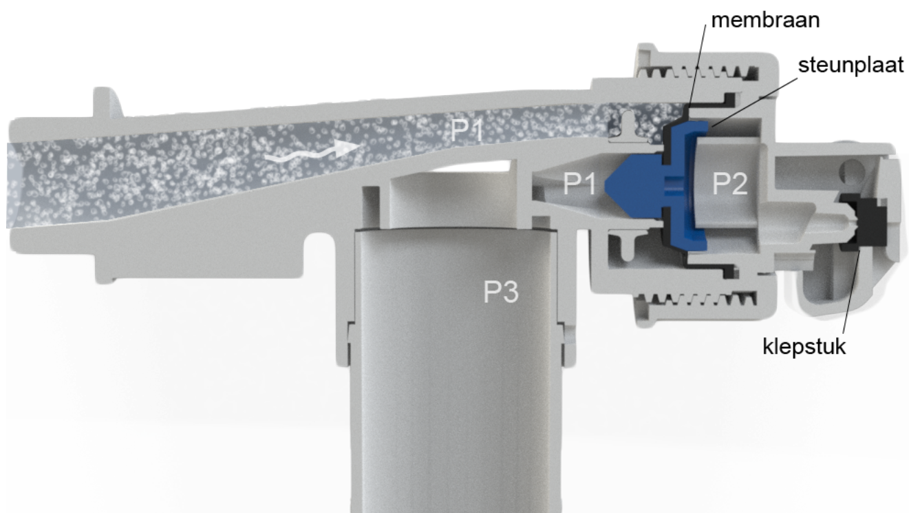
Fig 2 - kraan gesloten
