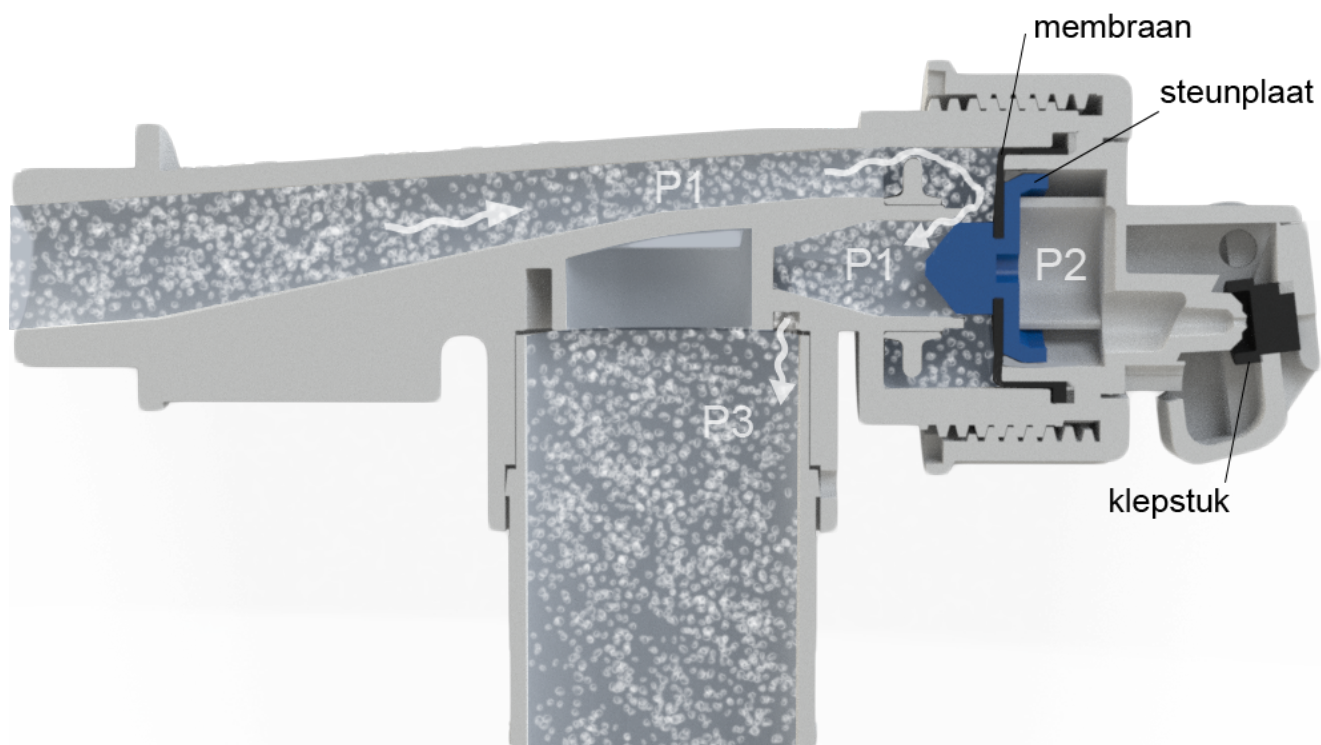
Fig 1 - kraan open
